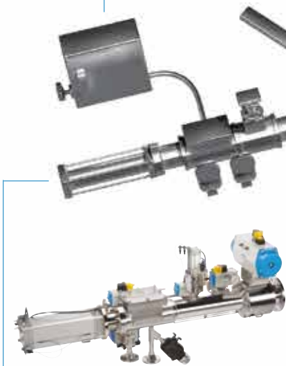
Sendsstation Manuelle Betätigung, vollautomatisierte Station für Einmolchsystem und Zweimolchsystem
